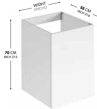
■ □ 1 DOOR ADDITIONAL UNIT MUEBLE AUXILIAR CON 1 PUERTA
