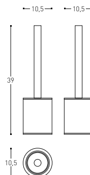
⊙◇ FREE STANDING TOILET BRUSH ESCOBILLERO SUELO
