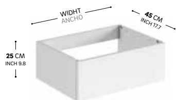
1 DRAWER CABINET FOR WASHBASIN MUEBLE CON 1 CAJÓN PARA LAVABO
