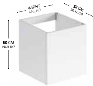
■ □ 1 DOOR ADDITIONAL UNIT MUEBLE AUXILIAR CON 1 PUERTA
