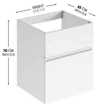
2 DRAWERS CABINET FOR WASHBASIN MUEBLE CON 2 CAJONES PARA LAVABO
