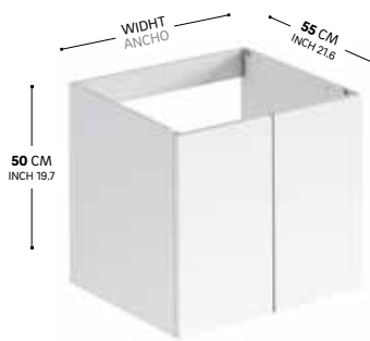
■ □ 2 DOORS ADDITIONAL UNIT MUEBLE AUXILIAR CON 2 PUERTAS
