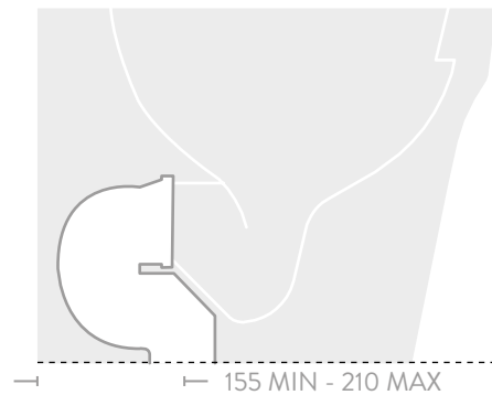
CURVA TECNICA TRASLATA ADJUSTABLE PIPE
