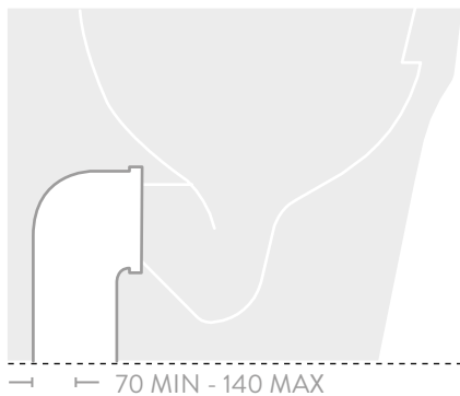
CURVA 90° REGOLABILE ADJUSTABLE 90° ELBOW
