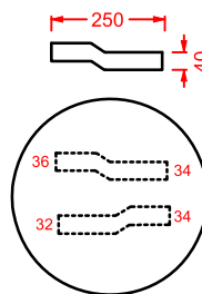
ART ACA035 CANNOTTO TRASLATO PER INGRESSO ACQUA +/- 2 CM
