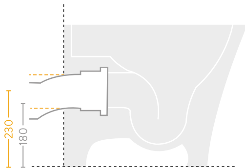
SCARICO A MURO WALL TRAP
